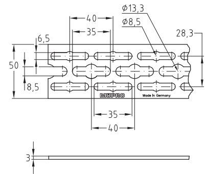
StaboFix® Направляющая
