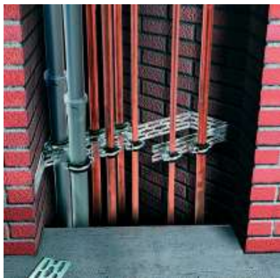
Монтаж в шахте: Сквозной монтаж с двумя хомутами MÜPRO и одной шпилькой MÜPRO M8 или M10 для крепления параллельных трубопроводов
